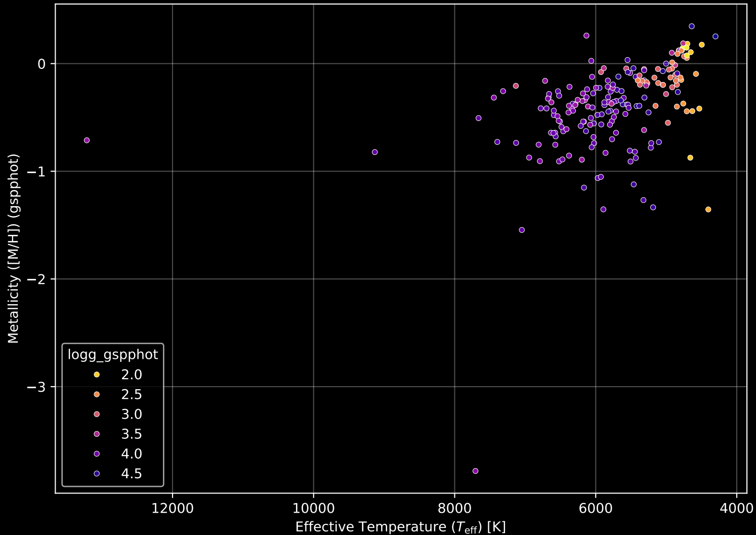
GALAH DR4 Field: [6588] Stellar Population Parameters (n= 190)
