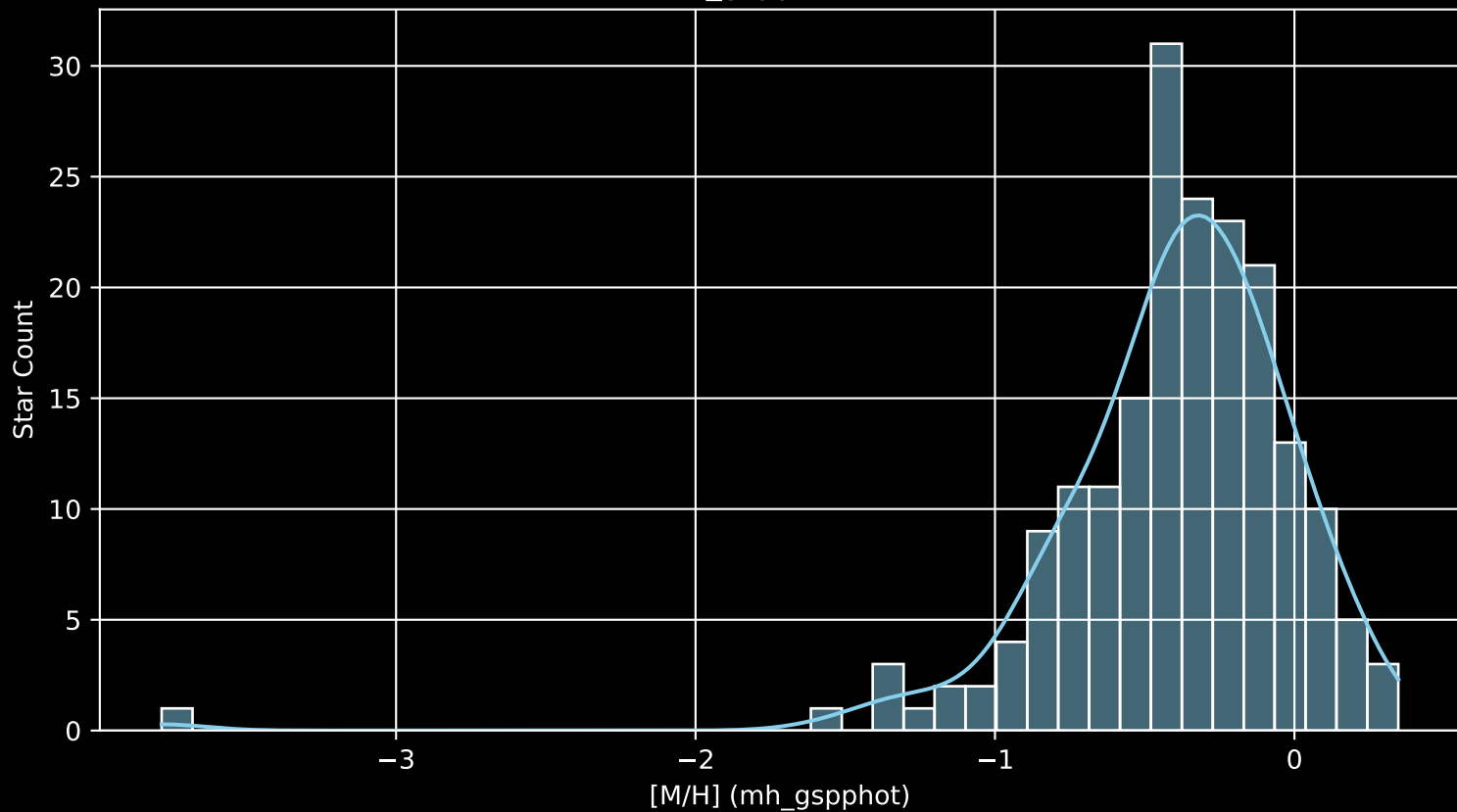
GALAH DR4 Field: [6588] [M/H] (mh_gspphot) (n= 190)
