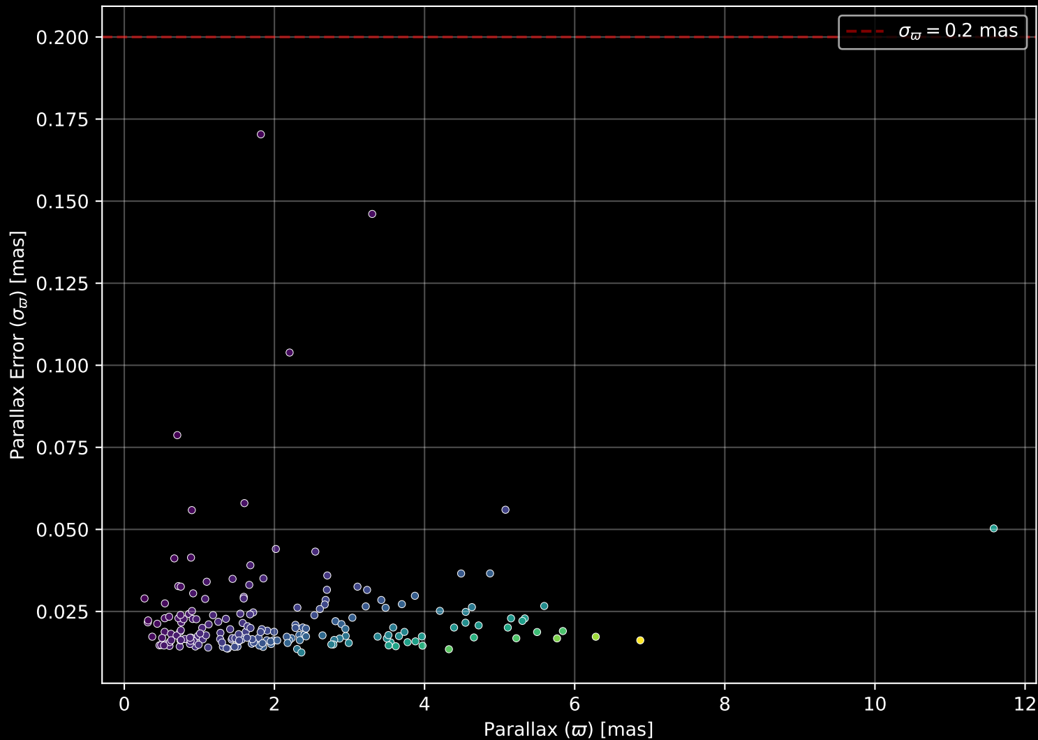
GALAH DR4 Field: [6588] Parallax Quality (n= 190)
