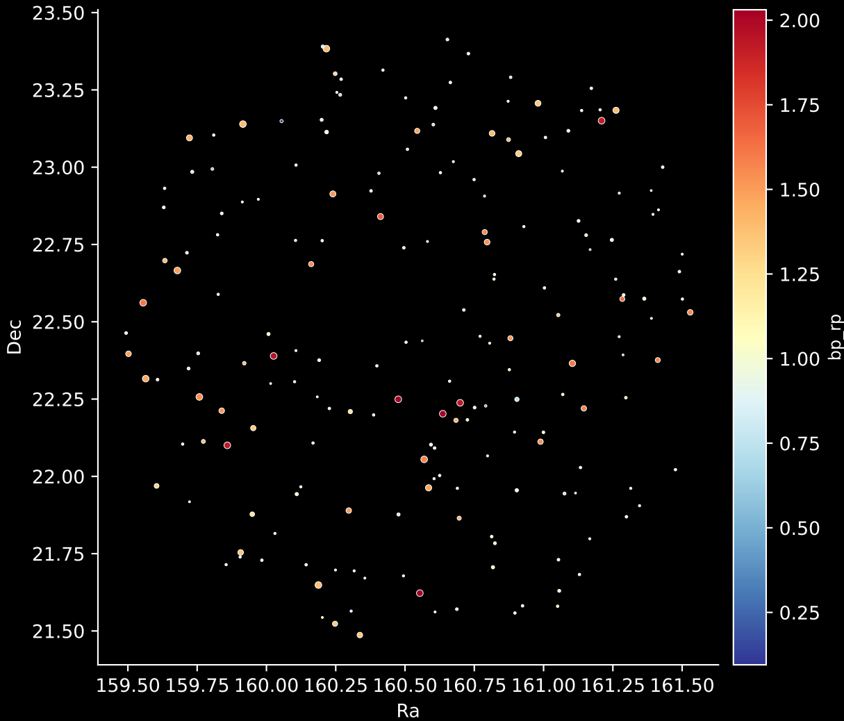
GALAH DR4 Field: [6588] Stars: 190
